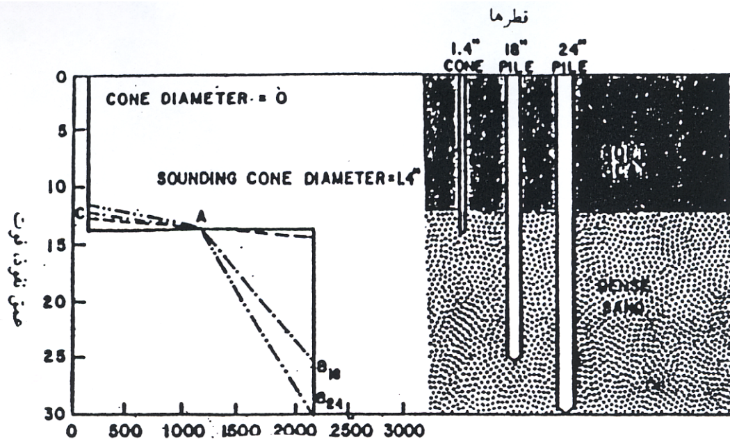
شکل ۲. اثر ابعاد قطر پترومتر در بسیج کامل مقاومت واحد کف شمع [۷] ————— شمع به قطر ۱۸ اینچ - - - - - شمع به قطر ۲۴ اینچ - · - · - · - پترومتر به قطر ۱ اینچ - · - · - · - پترومتر به قطر ۱/۴ اینچ
