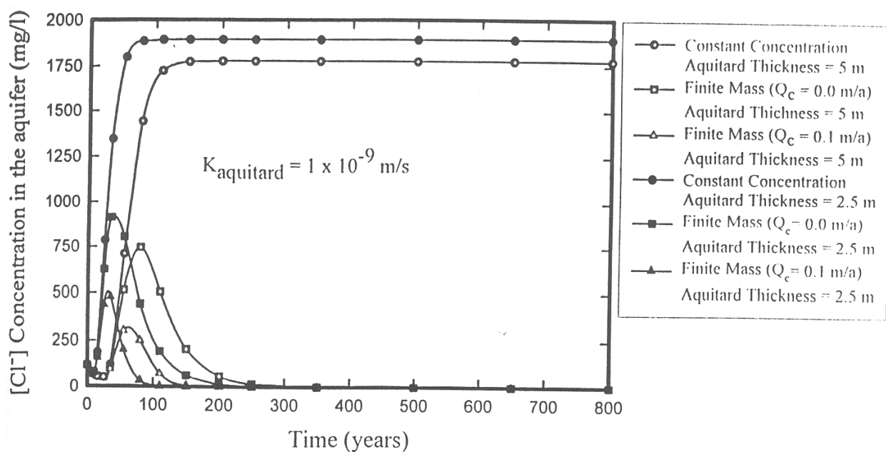
شکل ۸ - تغییرات غلظت یون کلر (Cl) در سفره آبدار نسبت به زمان در مدفن زباله با زهکشهای فرانسوی (گزینه دوم) در حالت طبیعی، (۱) تاثیر غلظت ثابت نسبت به غلظت یا جرم محدود در کف مدفن، (۲) تاثیر ضخامت لایه زمین طبیعی، K_{\text{aquitard}} = 1 \times 10^{-9} (m/s)، (۳) تاثیر میزان زهکشی شیرابه در کف مدفن.
