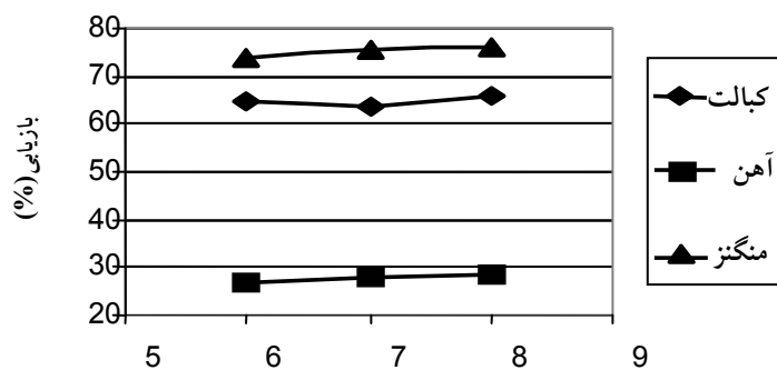
شکل ۵- اثر نسبت مایع به جامد بر بازیابی کبالت، آهن و منگنز
