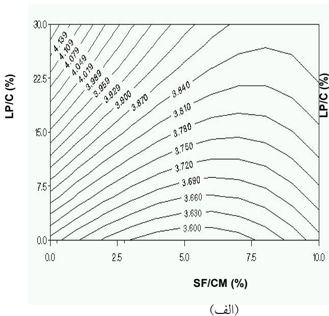
شکل ۶- منحنیهای هم پاسخ مربوط به CEF برای بتن با نسبت آب به مواد سیمانی ۰/۲۵؛ (الف) قیمت پودر سنگ آهک: ۰/۵۰؛ (ب) قیمت پودر سنگ آهک ۰/۲۰؛ قیمت سیمان
