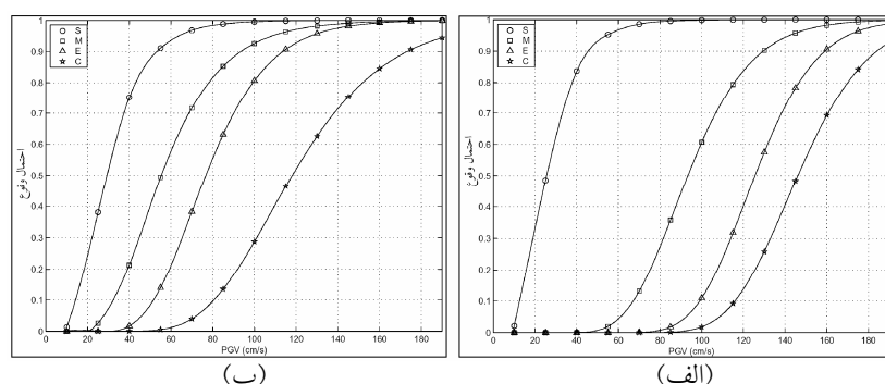
شکل ۲۶- منحنیهای شکنندگی لرزه‌ای حاصل از توابع IDDR و DIP_{P\&A} وابسته بر سرعت حداکثر زمین
