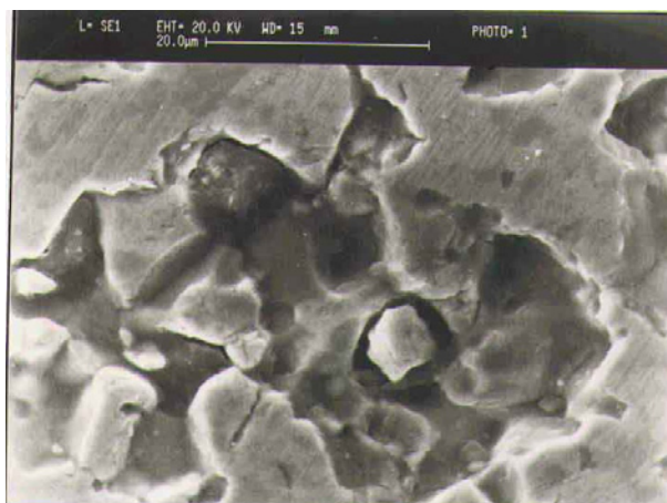
شکل ۷- تصویر SEM از الکترونیهای برگشتی نمونه Fe-10% Ti-3%C در حالت سرمایش و برگشت شده بعد از سائیده شدن به مسافت ۷۰۰ متر
