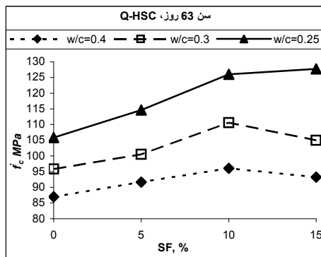
شکل ۱۰- مقاومت فشاری بتن شاهد با درشت دانه کوارتزیتی در مقابل درصدهای میکروسیلیس بعد از ۶۳ روز
