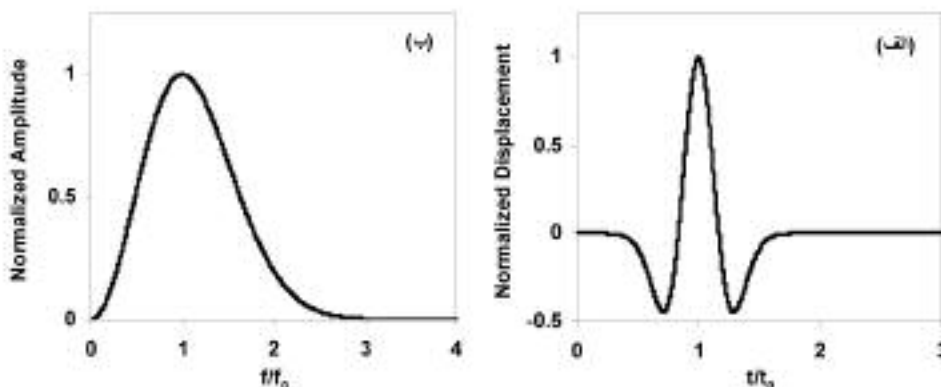
شکل ۴ - الف) تاریخچه زمانی و ب) طیف دامنه فوریه موج ریکر
