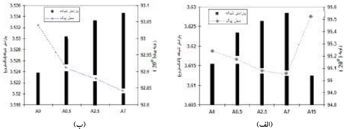
شکل ۲- تغییرات پارامتر شبکه و محل پیکها با پیشرفت آلیاژسازی مکانیکی الف) مس پیک (222). ب) نیکل پیک (311)
