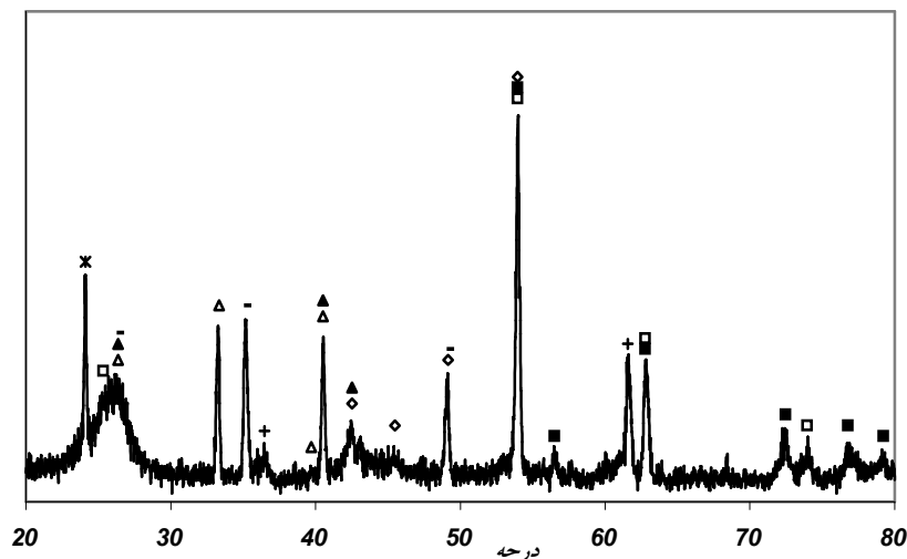
شکل ۶- الگوی پراش اشعه (x) باقی مانده آزمایش (TGA) نمونه آناتاز- کک بدون آسیابکاری (مخلوط سازی فیزیکی).
