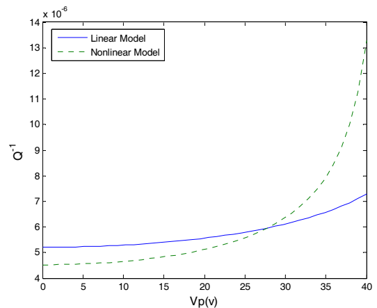
شکل ۳- تغییرات میرایی ترموالاستیک بر حسب ولتاژ در دو مدل خطی و غیرخطی در h = 5\mu\text{m}
