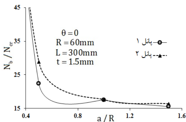
شکل ۱۱- تغییرات بار کمانش کششی بر حسب طول ترک در پانل با تکیه گاه گیردار
