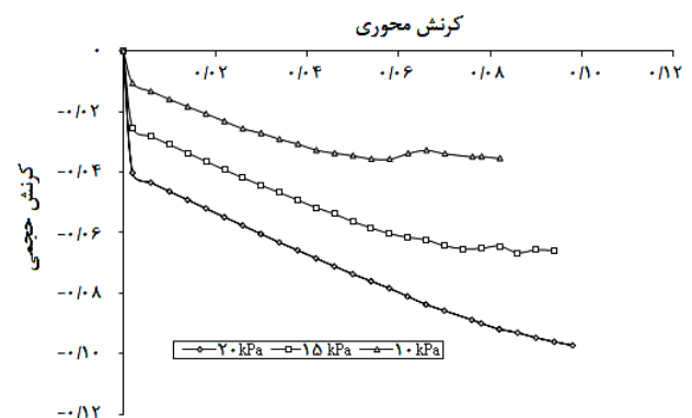
شکل ۳۷- نمودار تغییرات کرنش حجمی نسبت به کرنش محوری در نمونه با ضریب اصطکاک بین ذره‌ای 0/9 و Sr=20\%
