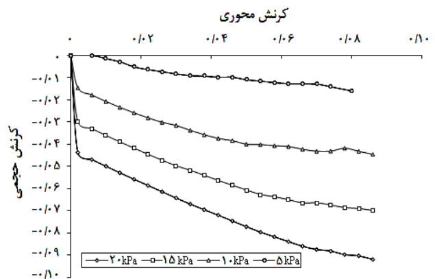
شکل ۳۶- نمودار کرنش حجمی نسبت به کرنش محوری در نمونه با ضریب اصطکاک بین ذره‌ای 0/5 و Sr=20\%
