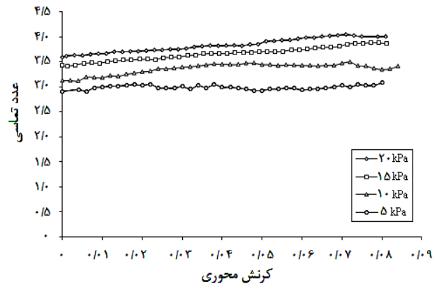
شکل ۳۵- نمودار تغییرات عدد تماسی نسبت به کرنش محوری در نمونه با ضریب اصطکاک 0/9 و در حالت خشک
