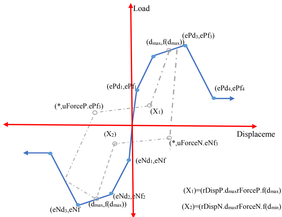
شکل ۸- مسیر رفت و برگشتی در مصالح Pinching4 [۲۰]
