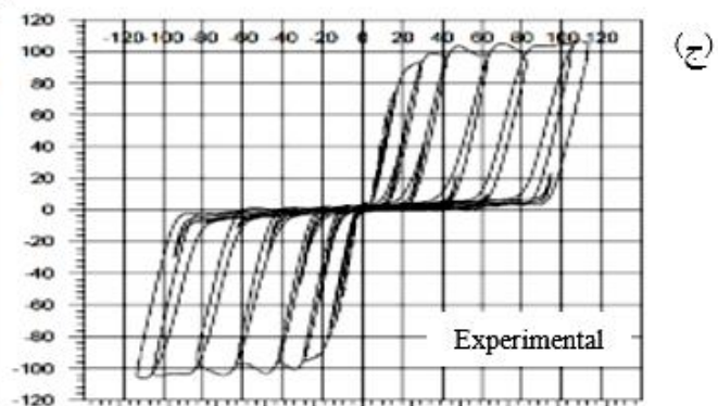
شکل ۱۲- نتایج صحت‌سنجی مدل‌های عددی قاب‌های با تسمه بادبندی تحت بار رفت و برگشتی با نتایج آزمایشگاهی: الف) نمونه 38A-C، ب) نمونه EAI حاتمی و همکاران [۱۴]، ج) نمونه 38A-C ولچو [۸]
