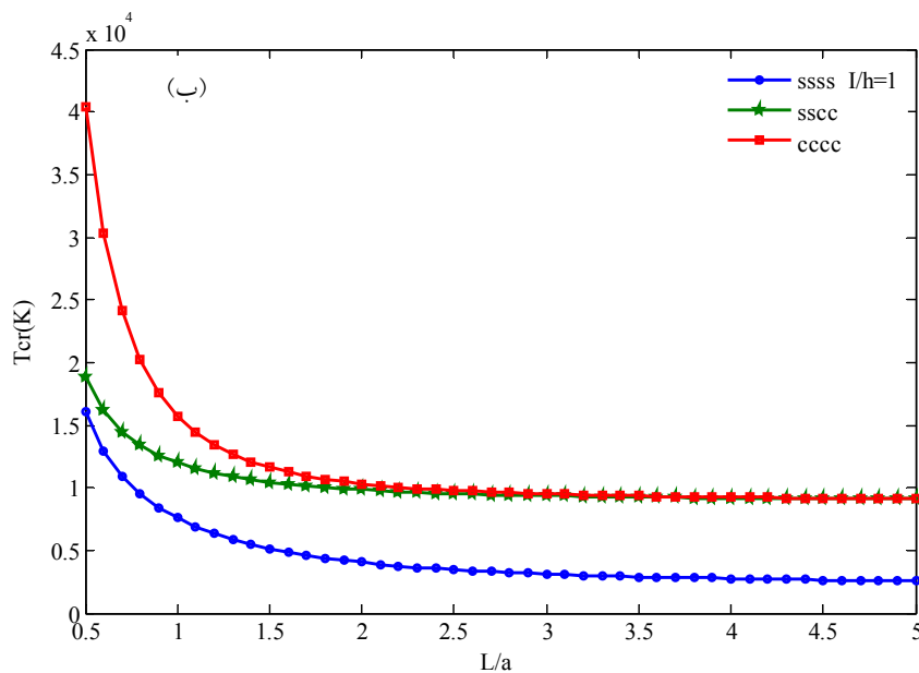
شکل ۲- تغییرات دمای بحرانی کماتش ورق برحسب نسبت طول به عرض در حالت توزیع یکنواخت دما برای نسبت پارامتر مقیاس طول به ضخامت برابر با: الف) صفر و ب) یک
