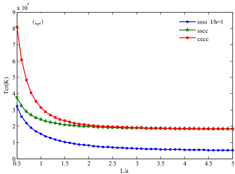
شکل ۳- تغییرات دمای بحرانی کمانش ورق بر حسب نسبت طول به عرض در حالت توزیع خطی دما برای نسبت پارامتر مقیاس طول به ضخامت برابر با: الف) صفر و ب) یک
