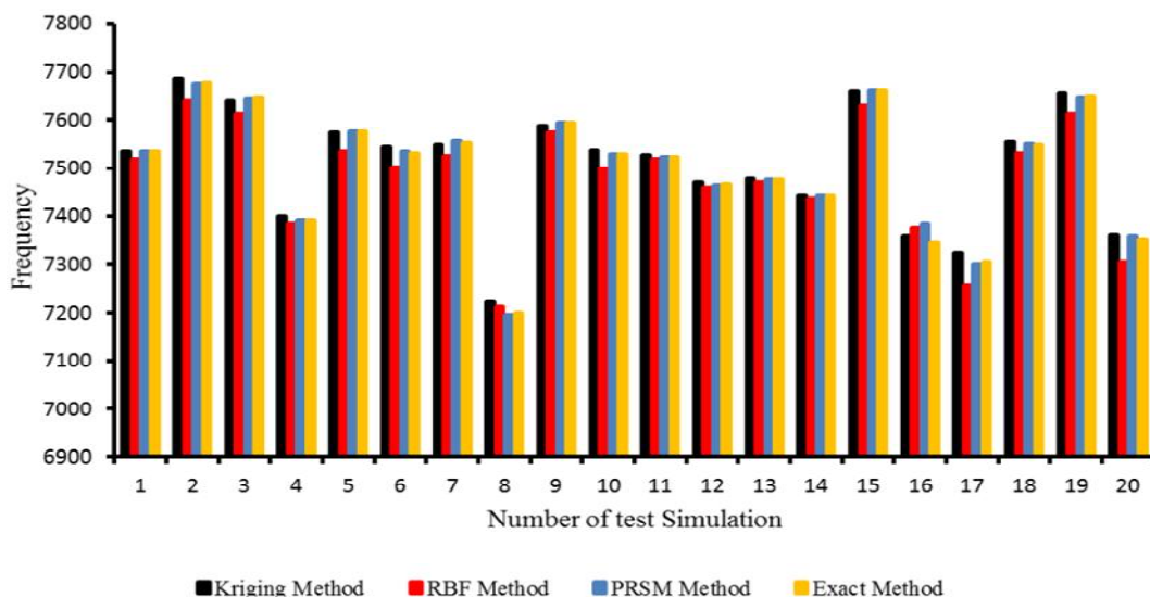
شکل ۵- مقایسه بین بسامدهای مود اول حاصل شده از ارتعاش آزاد صفحه سه لایه FGME با استفاده از روش‌های پیش‌بینی پاسخ و روش حل سه‌بعدی
