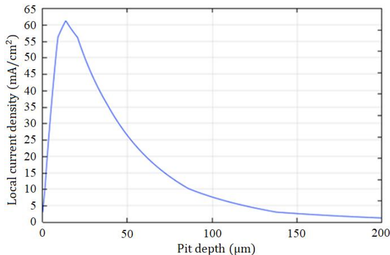
شکل ۱۸- تغییرات چگالی جریان داخل حفره برای پتانسیل 350 \text{ mVsCE}
