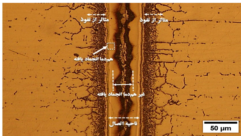
شکل ۵- ناحیه اتصال فولاد زنگ نزن ۳۰۴ L درشت دانه در زمان ۵ دقیقه و دمای ۱۰۵۰°C
