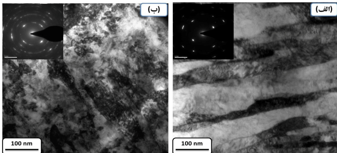
شکل ۴-تصاویر میکروسکوپی الکترونی عبوری از ریزساختار فولاد زنگ نزن ۳۰۴ L پس از ۸۰٪ نورد سرد
