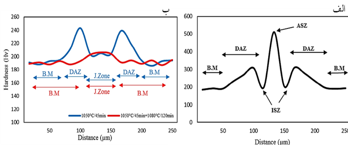
شکل 8. پروفیل سختی اتصال مشابه اینکونل 600 (الف) دمای 1050 و زمان 5 دقیقه و (ب) اتصالات همگن سازی شده.
