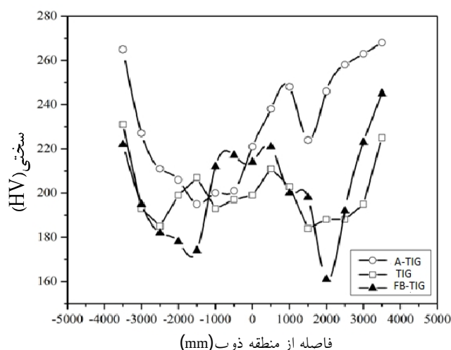
شکل ۱۲- پروفیل سختی در روش‌های TIG, A-TIG و FB-TIG
