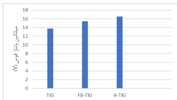
شکل ۱۱- نمودار تغییرات میانگین ولتاژ در روش‌های TIG, A-TIG و FB-TIG
