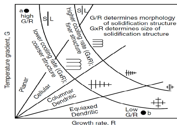
شکل ۹- نحوه تغییرات ریزساختار انجمادی با گرادین دمای و سرعت انجماد [۹].
