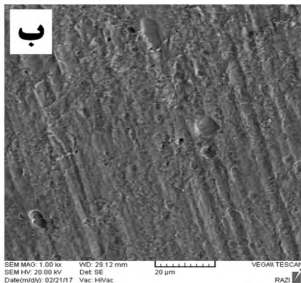
شکل 6- تصاویر میکروسکوپ الکترونی روبشی از سازوکار خوردگی فلز جوش ایجاد شده با حرارت ورودی: الف) ۱۲/۶ kJ/mm ، ب) ۳۷/۸ kJ/mm
