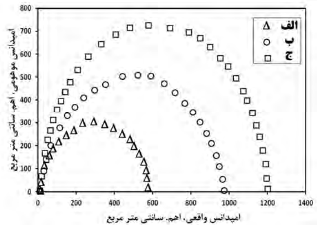
شکل 5- نمودار نایکویست مربوط به آزمایش طیف سنجی امپدانس الکتروشیمیایی با حداقل سه بار تکرارپذیری برای فلز جوش ایجاد شده با حرارت ورودی: الف) ۱۲/۶ kJ/mm، ب) ۱۸/۹ kJ/mm، ج) ۳۷/۸ kJ/mm.
