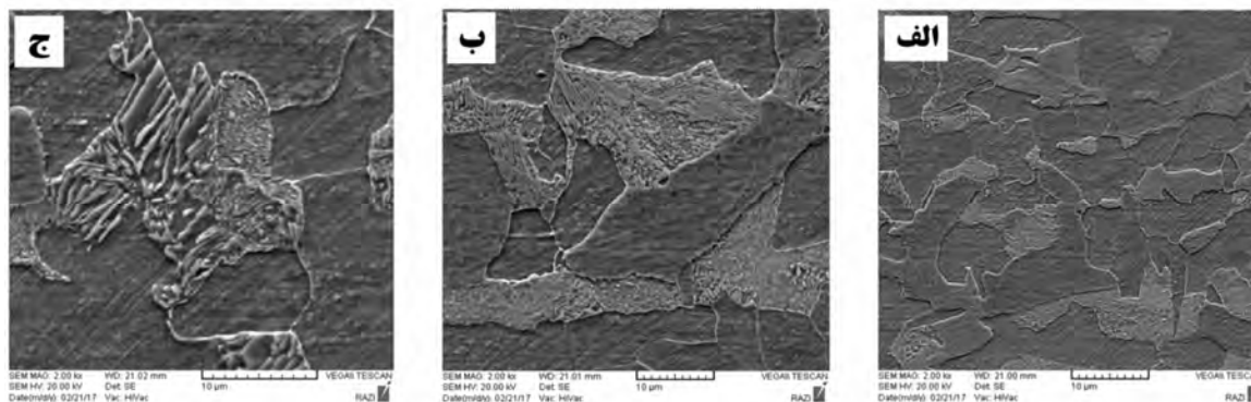
شکل 2- تصویر میکروسکوپ الکترونی روبشی از فلز جوش ایجاد شده با حرارت ورودی: (الف) 12,6 kJ/mm ، (ب) 18,9kJ/mm ، (ج) 37,8kJ/mm.
