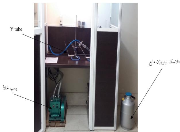
شکل 1- شمایی از مونتاژ تهیه شده برای انجام آزمایش اندازه‌گیری هیدروژن جوش
