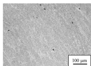
شکل 7- تصویر میکروسکوپی نوری از ریزساختار فلز پایه در دو بزرگنمایی متفاوت (اچ شده با محلول نایتال 2%)
