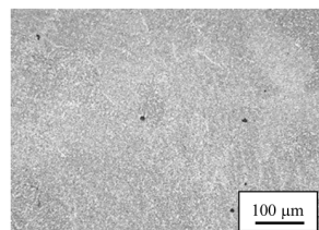
شکل 8 - تصاویر میکروسکوپی نوری با بزرگنمایی برابر از ریزساختار منطقه جوش حاصل از جوشکاری. اعداد زیر هر تصویر مربوط به شرایط اعمال شده طبق جدول 6 می‌باشد. (اچ شده با محلول نایتال 2%)
