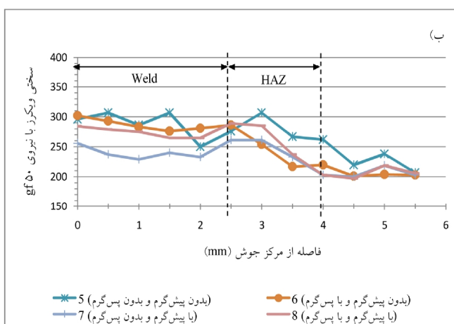
شکل 10- نتایج آزمایش میکروسختی به روش ویکرز با نیروی 50 gf به صورت یک پروفیل از وسط جوش تا فلز پایه. الف) نمونه های جوشکاری شده با الکتروکد سلولزی E8010-P1. ب) نمونه های جوشکاری شده با الکتروکد کم هیدروژن E8018-G.
