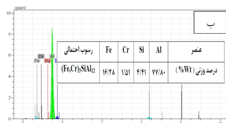
شکل ۵- تصویر میکروسکوپ نوری و آنالیز EDS رسوبات فلز پایه آلومینوم (۶۰۶۱: الف) تصویر میکروسکوپ نوری، ب) آنالیز EDS رسوبات.
