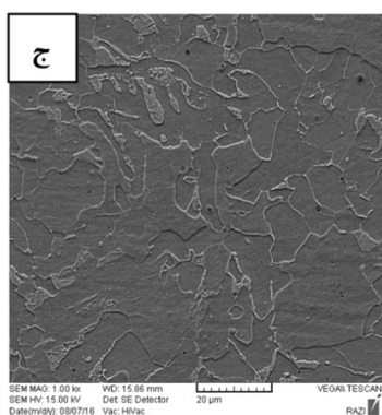
شکل 6-الف) تصاویر میکروسکوپی ناحیه متأثر از حرارت، ب) ریشه جوش و ج) منطقه جوش در موقعیت 6-7/30
