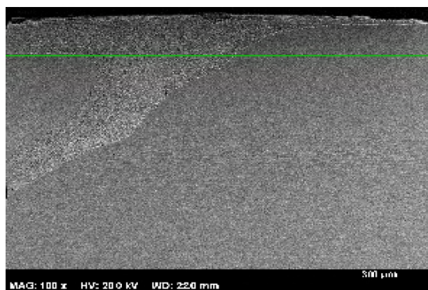
شکل 20- تصویر میکروسکوپ الکترونی و توزیع عناصر در آنالیز خطی در نمونه (a) از سمت فولاد 316 L به طرف ناحیه همزده.
