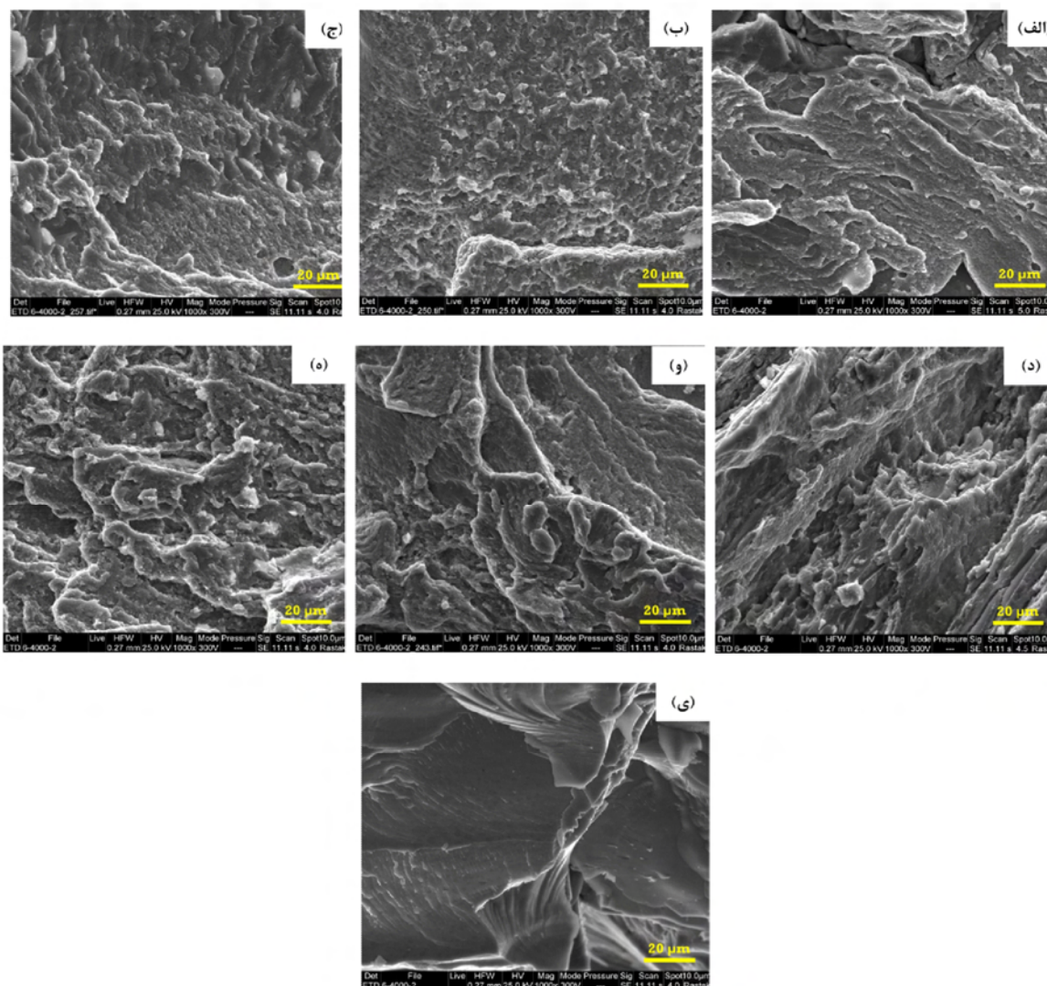
شکل ۸- تصویر میکروسکوپ الکترونی از سطح شکست نمونه:
