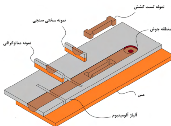
شکل ۳- شماتیک فرایند به همراه نمونه های برش خورده جهت تست کشش، سختی سنجی و متالوگرافی
