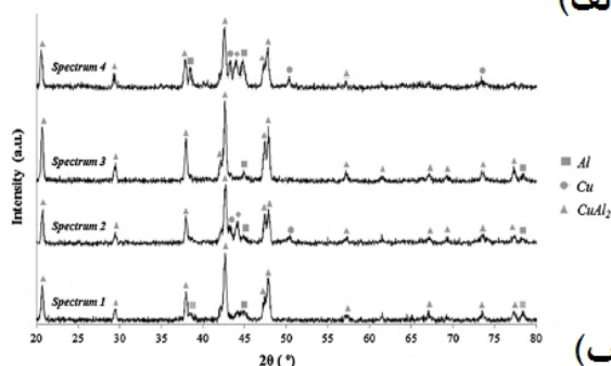
شکل ۱۱- نمونه آنالیز پراش پرتو ایکس از منطقه اغتشاش که با ابزار (الف) ساده و (ب) رزوه ای جوشکاری شده اند
