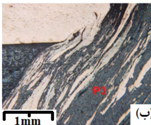
شکل ۹- ساختار لایه ای شکل گرفته با ابزار (الف) رزوه ای و (ب) ساده
