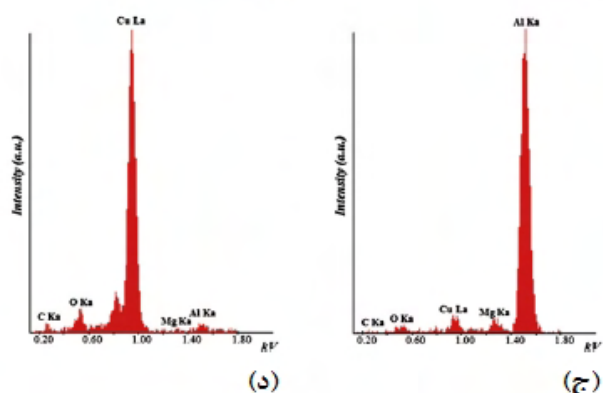
شکل ۱۰- نمونه آنالیز EDS از نقاط ساختارهای لایه ای که با ابزار (الف) و (ب) ساده و (ج) و (د) رزوه ای جوشکاری شده اند
