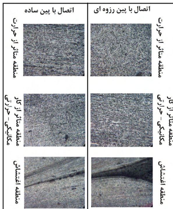
شکل ۷-نواحی مختلف جوشکاری شده فلز آلومینیوم ۶۰۶۵
