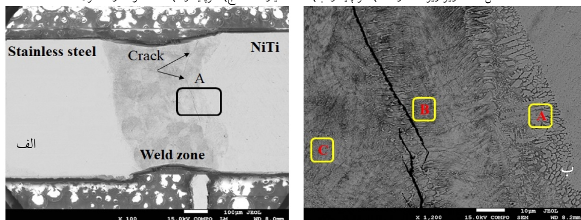
شکل 7- تصاویر SEM الف) ترک‌های موجود آمده در مرز مشترک ذوب و فلز پایه NiTi و ب) منطقه مشخص شده در تصویر الف) و نقاط آنالیز EDS.
