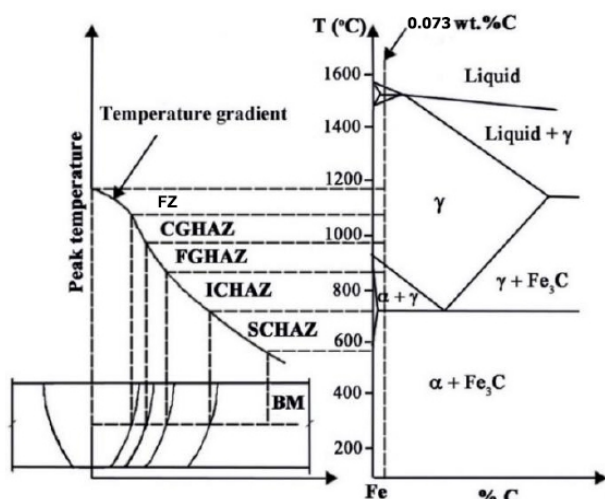
شکل 8- شماتیک نواحی نمودار تعادلی آهن کربن و ارتباط آن با سطح مقطع جوش فولاد های دو فاز
