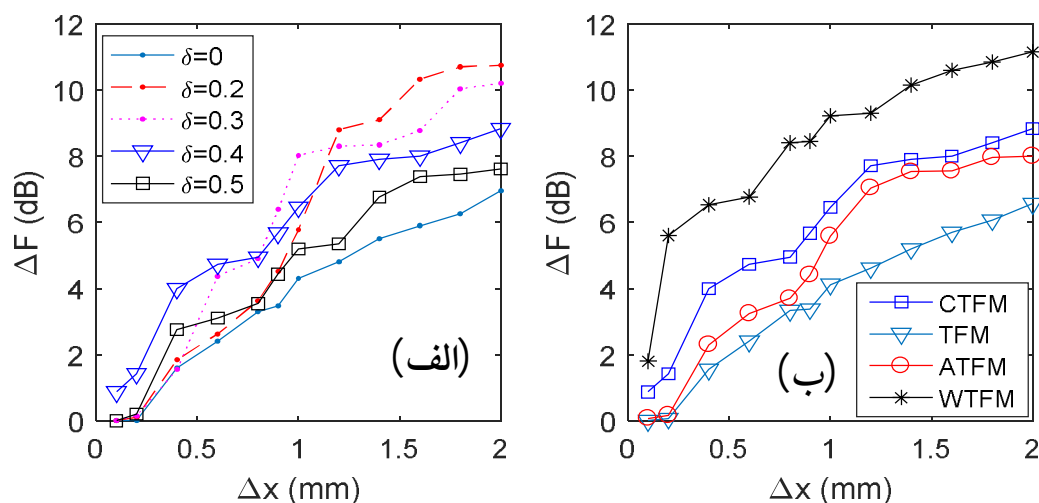
شکل 11- نمودار تابع \Delta F بر حسب فاصله بین دو نقطه بازتابنده مجاور: الف) نمودار تابع \Delta F در روش CTFM برای \delta های مختلف و ب) مقایسه تابع \Delta F برای CTFM با \delta = 0.4 و TFM، ATFM و WTFM
