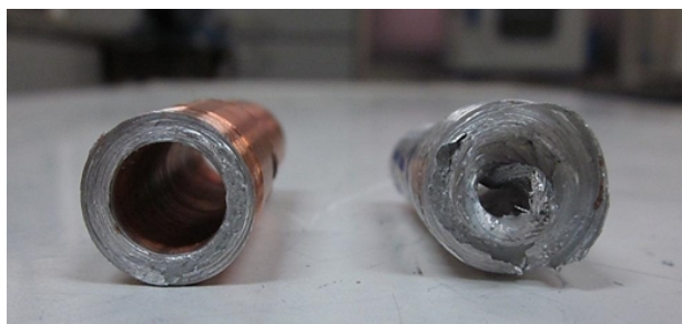
شکل 15- نحوه شکست نمونه‌های گروه دوم
