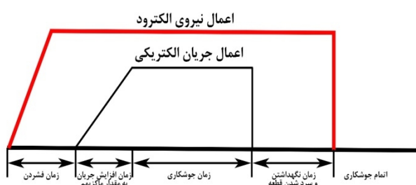
شکل 1- نحوه زمان بندی اعمال نیروی الکتروتودها و جریان الکتریکی جهت انجام جوشکاری مقاومتی نقطه‌ای.
