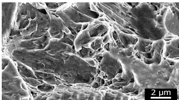
شکل 3- تصویر SEM از سطح مقطع شکست نمونه ضربه در آزمایش شماره 9
