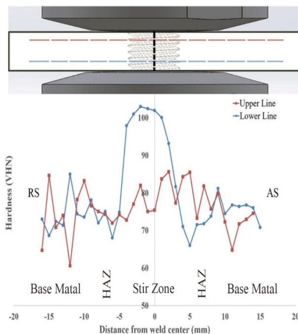
شکل 8- پروفیل سختی سطح مقطع عرضی جوش.
