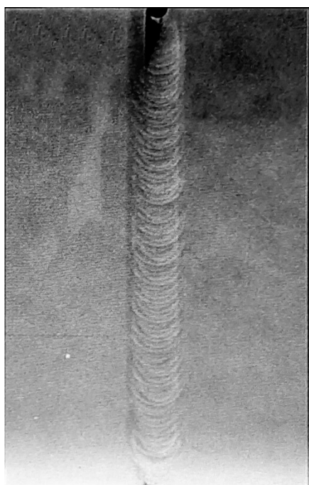
شکل 5 - رادیوگراف دیجیتال.
