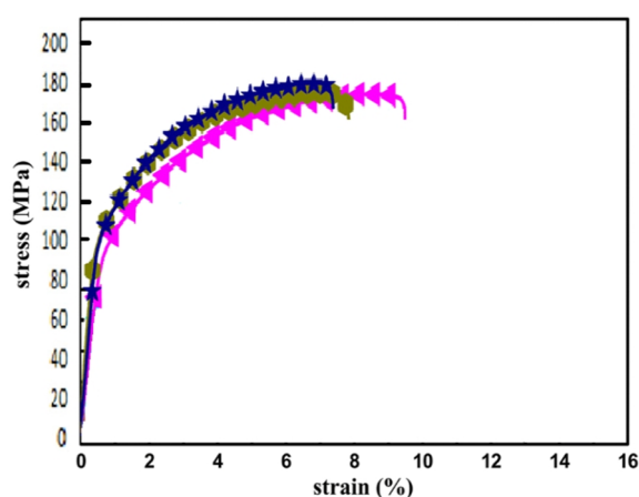
شکل 10- نمودار تنش-کرنش آلیاژ AZ91Cp (شرایط نمونه 2) جوشکاری شده تحت دمای پیشگرم 523K و شدت جریان 110 A (3 مرتبه تکرار)
