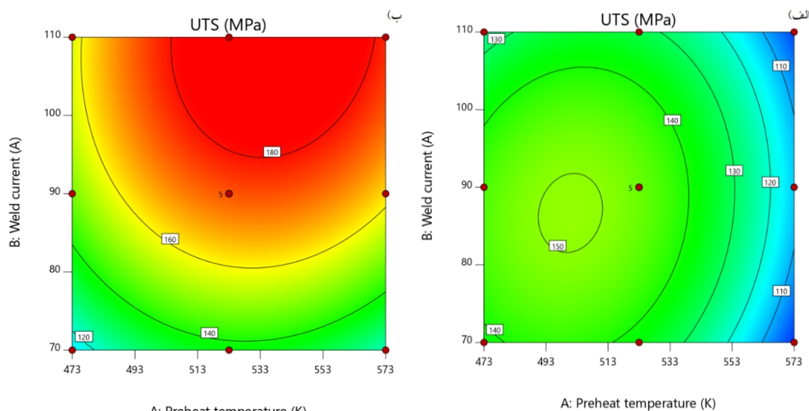
شکل 9- نمودارهای تراز برای استحکام نهایی کششی الف- شرایط نمونه 1؛ ب- شرایط نمونه 2. A: Preheat temperature (K) B: Weld current (A)
