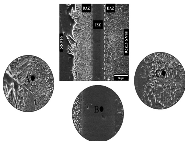
شکل 4- تصویر میکروسکوپ الکترونی روبشی (SEM) اتصال انجام شده در دمای 1150 درجه سانتی‌گراد و زمان 5 دقیقه
