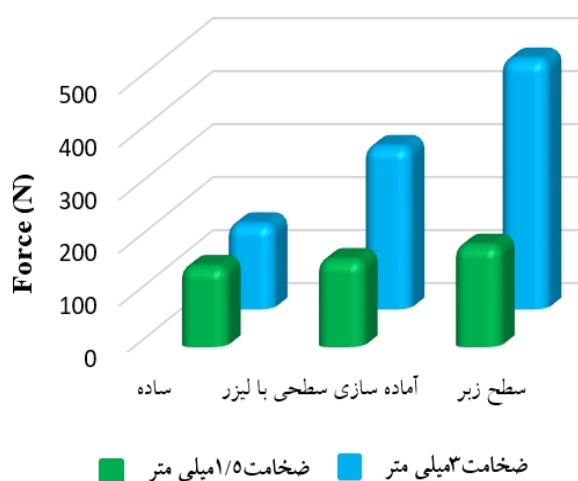
شکل 9- مقایسه استحکام کششی نمونه ها
