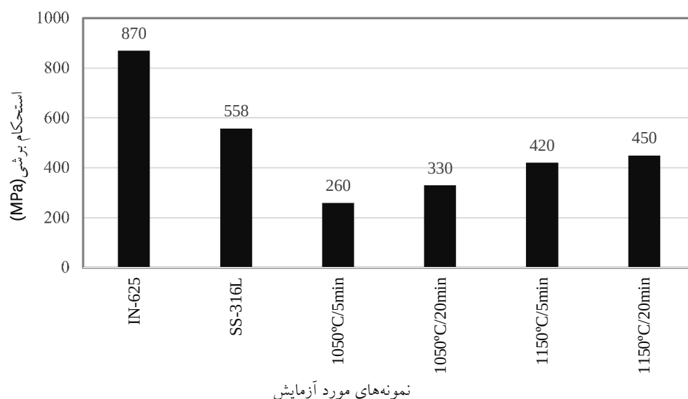
شکل 10- تاثیر شرایط اتصال دهی بر استحکام برشی نمونه‌های اتصال داده شده.
