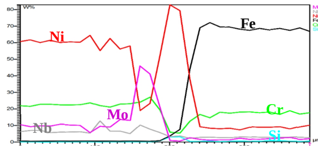
شکل 4- پروفایل توزیع عناصر آلیاژی در امتداد موضع اتصال مجموعه SS-316L/BNi3/IN-625 اتصال داده شده در شرایط: الف - 1150 °C/5 min، ب - 1150 °C/20 min.
