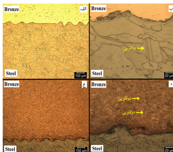
شکل 2- تصویر ریزساختار زمینه برنز (فلز پرنده) و فولاد (فلز پایه) و
