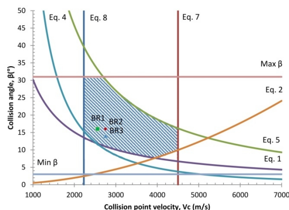
شکل 1- پنجره جوشکاری انفجاری محاسبه شده برای برنز و فولاد با استفاده از معادلات (1-8).
