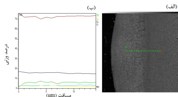
شکل 12- الف - طیف‌سنجی خطی تفکیک انرژی از روکش فولاد زنگ‌زن 17-4PH به سمت زیرلایه
