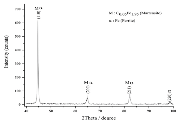
شکل 11- الگوی پراش پرتو ایکس از زیرلایه.
