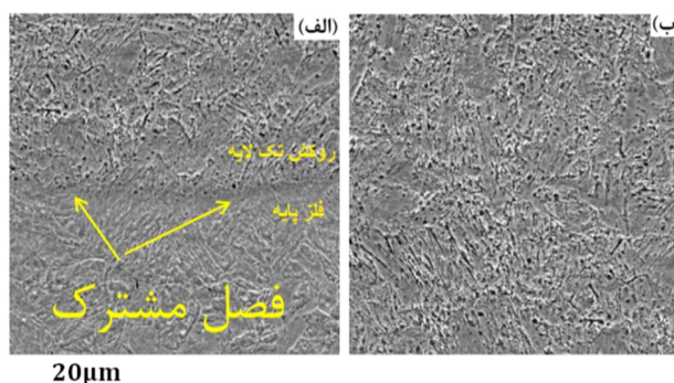
شکل 9- الف- تصویر میکروسکپی الکترونی روبشی از فصل مشترک روکش فولاد زنگ‌نزن 17-4PH با زیرلایه ب- تصویر میکروسکپی الکترونی روبشی از ریزساختار روکش فولاد زنگ‌نزن 17-4PH.
