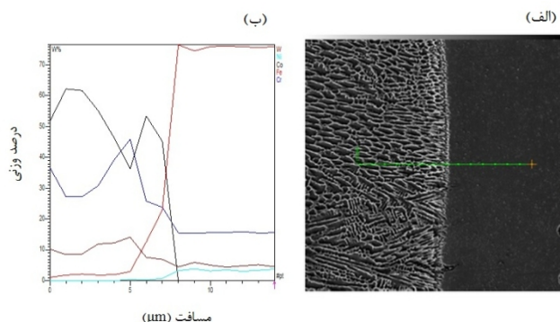
شکل 8- تصویر میکروسکوپی الکترونی رویشی از منطقه متاثر از حرارت در فولاد زنگ نزن 4PH-17.
