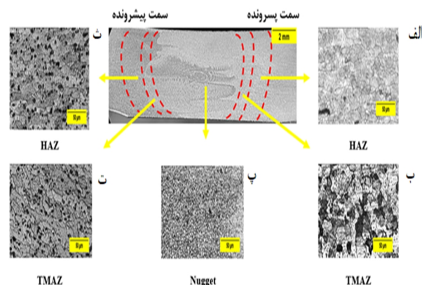
شکل 10- نمونه شماره 8 (سرعت جرخشی 1000 rpm و سرعت پیشروی
