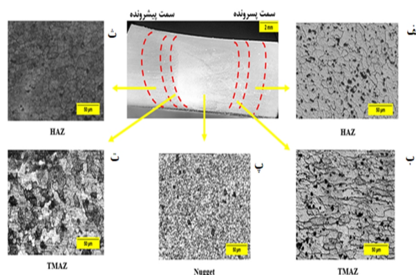
شکل 9- مقطع عرضی نمونه شماره 7 (سرعت چرخشی 600 و سرعت انتقالی 90 mm/min) و تصویر میکروسکوپی منطقه، الف - ناحیه متأثر از حرارت در سمت پسرونده، ب - ناحیه متأثر از عملیات ترمومکانیکی در سمت پسرونده،
