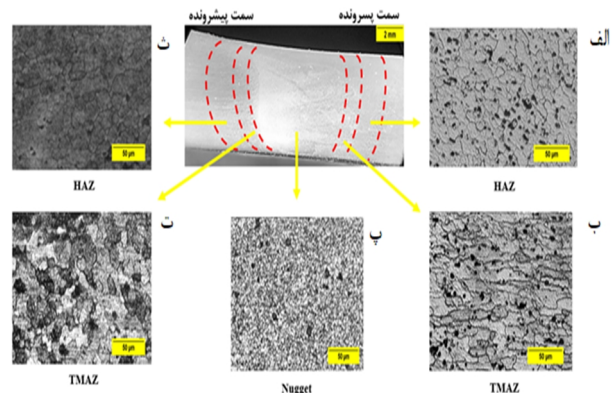
شکل 9- مقطع عرضی نمونه شماره 7 (سرعت چرخشی 600 و سرعت انتقالی 90 mm/min) و تصویر میکروسکوپی منطقه، الف- ناحیه متأثر از حرارت در سمت پیشرونده، ب- ناحیه متأثر از حرارت در سمت پسرونده، پسروده،
