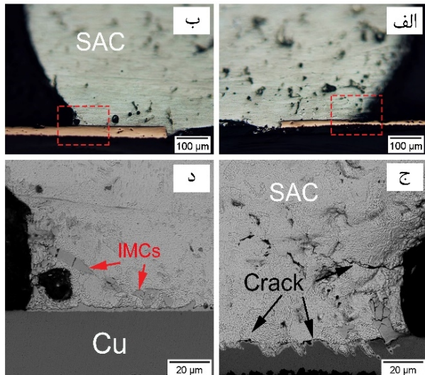
شکل 5- تصاویر ریزساختاری از سمت کاتد الف و ج- و آند ب و د- آلیاژ لحیم غیر کامپوزیتی بعد از گذشت 1135 ساعت از زمان آزمون مهاجرت الکترونی: الف و ب- تصاویر میکروسکپ نوری، ج و د- تصاویر میکروسکپ الکترونی.
