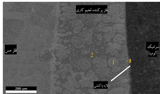
شکل 12- تصویر میکروسکوپی الکترونی روبشی از اتصال Al_2O_3/Cu با فلزپرکننده Ag-Cu-Ti-Sn-3.5Zr .
