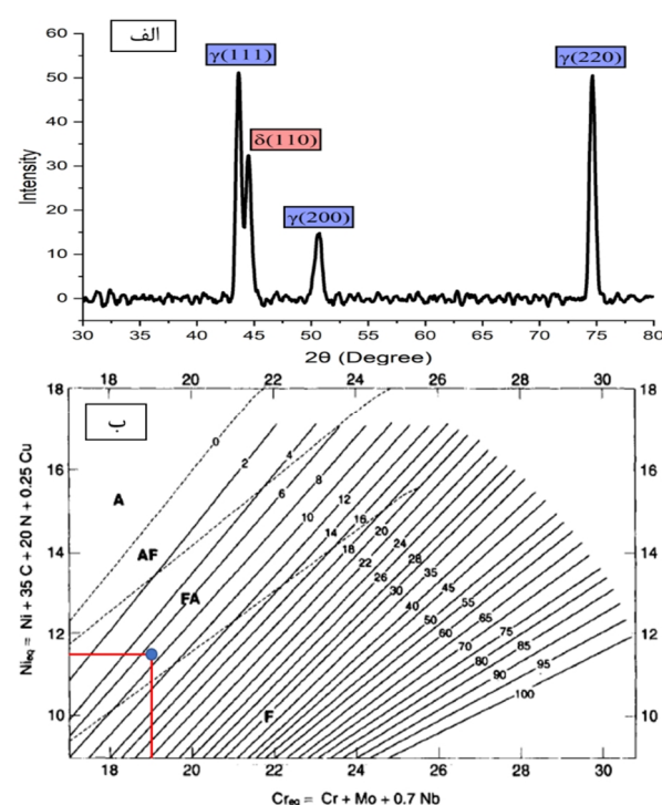
شکل 11-الف - الگوی از پراش پرتو ایکس فلز جوش فولاد 316 L ب- نمودار WRC-1992 برای تعیین حالت انجماد و تخمین میزان فریت جوش [20].
