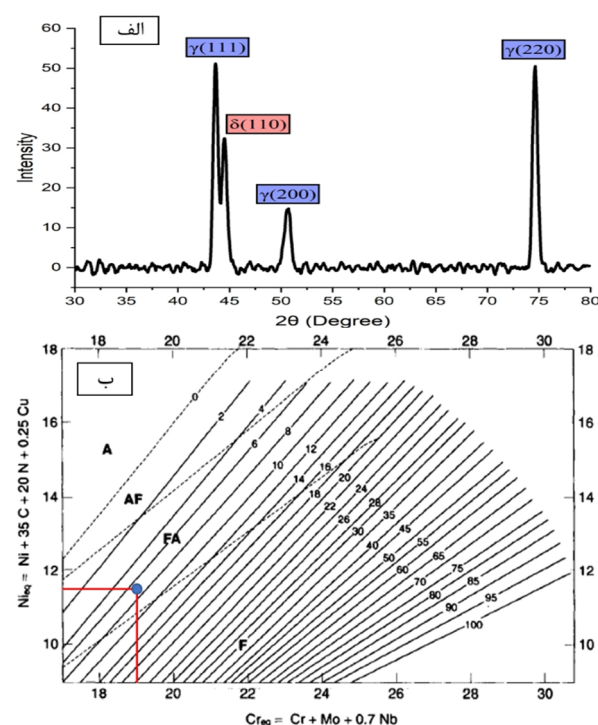
شکل 11-الف - الگوی از پراش پرتو ایکس فلز جوش فولاد 316 L
