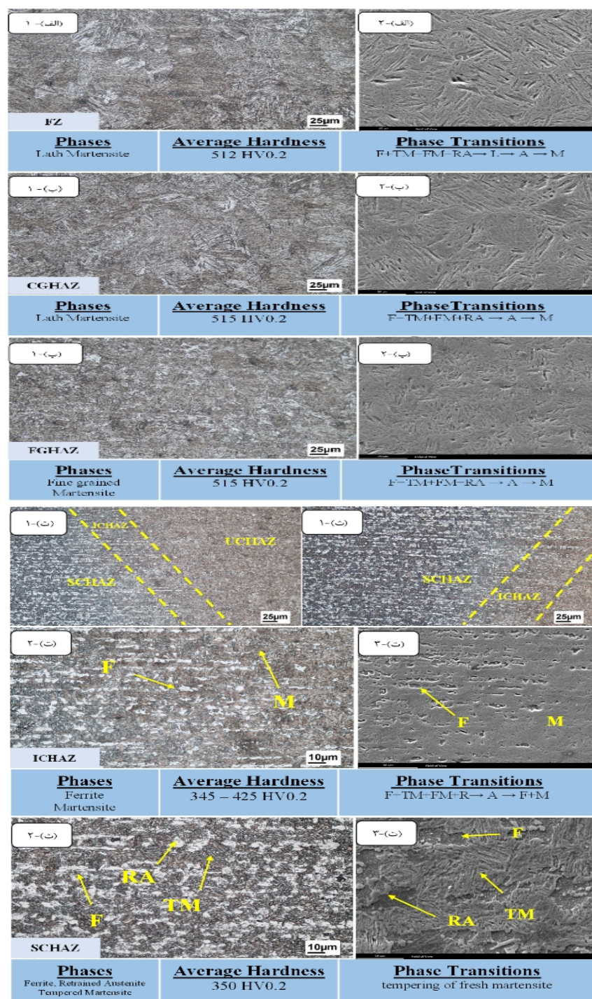
شکل 10- الف - ریزساختار دکمه جوش تصویربرداری شد با (1) LOM، (2) SEM. ب- ریزساختار منطقه متأثر از حرارت درشت دانه گرفته شده با (1) LOM، (2) SEM. پ- ریزساختار منطقه متأثر از حرارت ریز دانه گرفته شده با (1) LOM، (2) SEM. ت- 1- تفکیک مناطق متأثر از حرارت میانی، پایینی و فوق بحرانی. 2- ریزساختار منطقه متأثر از حرارت میانی گرفته شده با LOM، 3- گرفته شده با SEM. ث- 1- تفکیک منطقه متأثر از حرارت میانی و پایینی، 2- ریزساختار منطقه متأثر از حرارت پایینی گرفته شده با LOM، 3- گرفته شده با SEM: F فریت، M: مارتنزیت، FM: مارتنزیت تازه، TM: مارتنزیت معتدل، A: آستنیت، RA: آستنیت باقی مانده.
