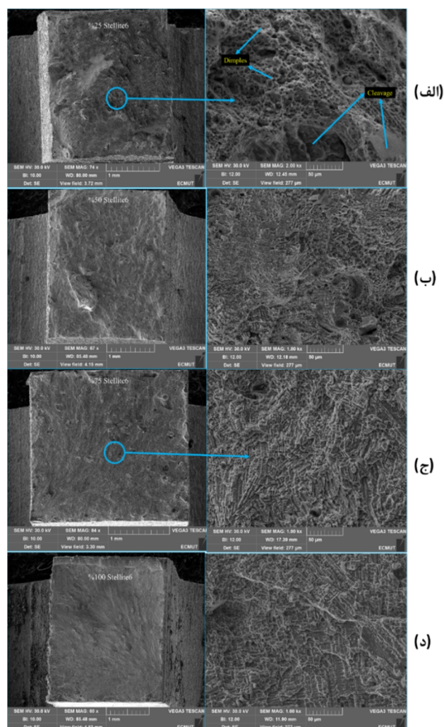
شکل 13- تصاویر میکروسکوپ الکترونی از مقاطع شکست ترکیبات
