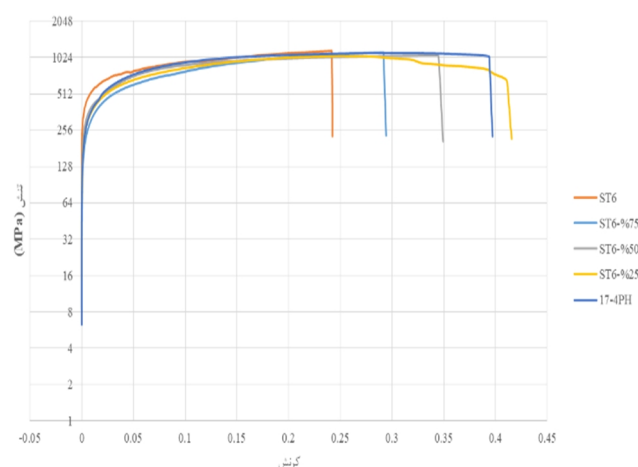
شکل 11- نمودار تنش- کرنش برای نمونه های ساخته شده با درصد ترکیبی برای 17-4PH و Stellite6 به ترتیب 0-100، 25-75، 50-50، 75-25 و 100-0
