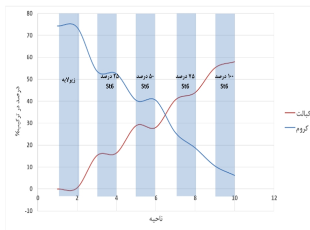
شکل 8- تغییرات عناصر آهن و کربالت بر حسب نواحی مختلف رسوب‌نشانی.
